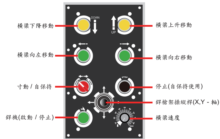
TEA-2020BP/TC 使用
