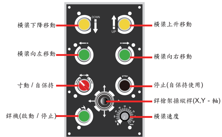
TEA-2020BP/TC 使用
