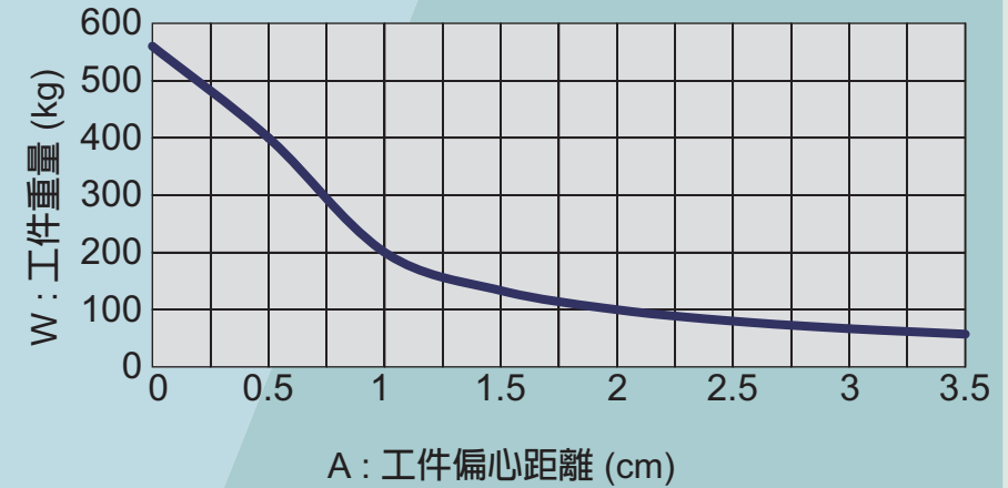
POSD120D 旋轉荷重偏心距離表
