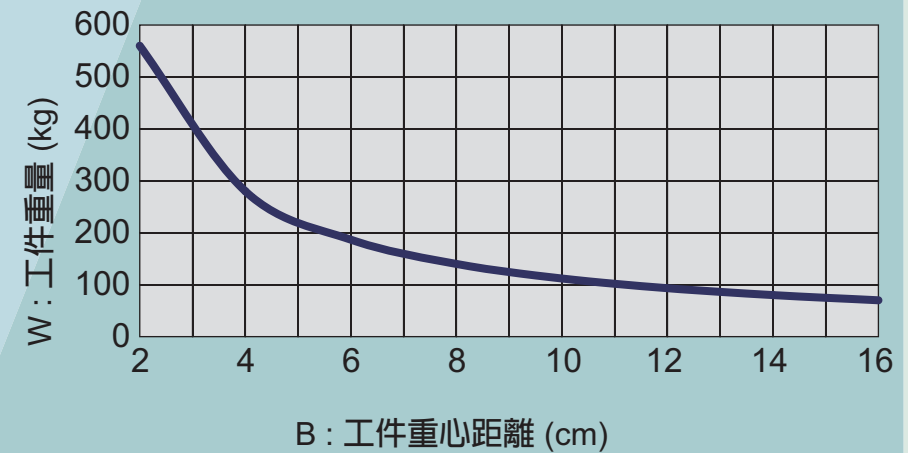
POSD120D 盤面傾斜重心高度表
