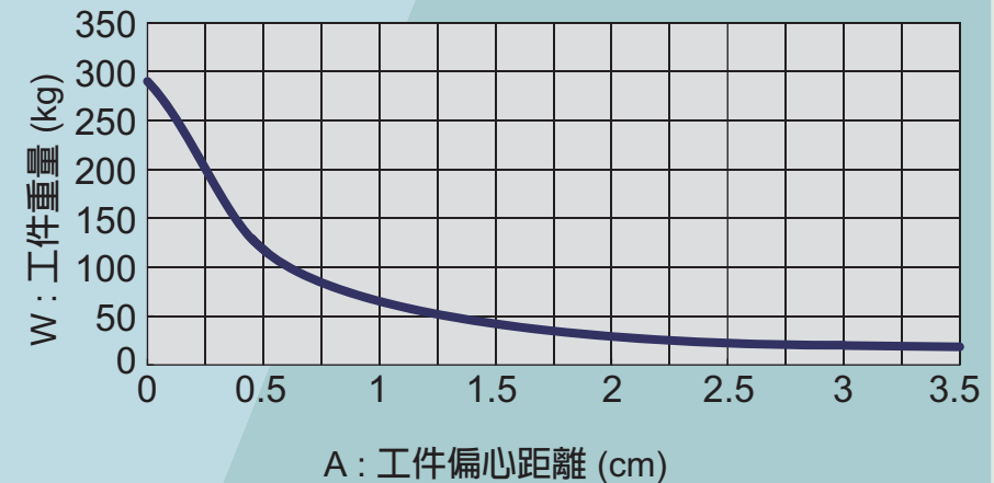
MPOS1C 旋轉荷重偏心距離表
