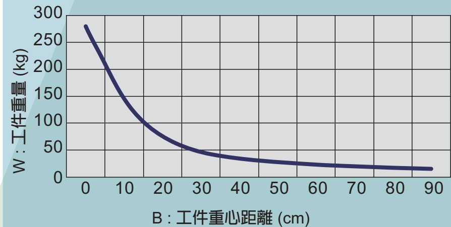
MPOS1C 盤面傾斜重心高度表
